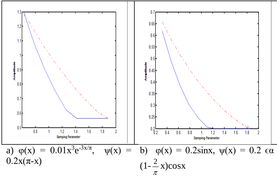
Fig.4. Amplitude vs. damping parameters \alpha
